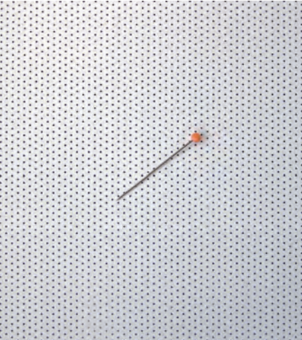
Lochbild im Massstab 1:1: finest 1.8/1.8/0.5 mm , offene Fläche 6.1%, 308.642 Löcher/m 2
