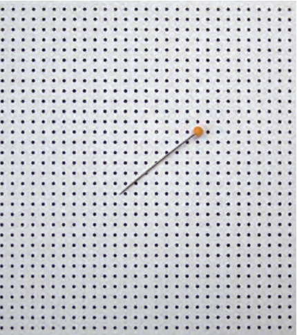
Lochbild im Massstab 1:1: classic 3/3/1 mm , offene Fläche 8.7%, 111.111 Löcher/m 2
